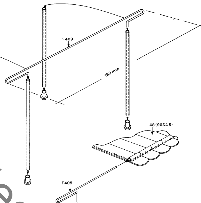
FIG. 8: MARQUESINA Y HERRAJES PARA EL PALO
