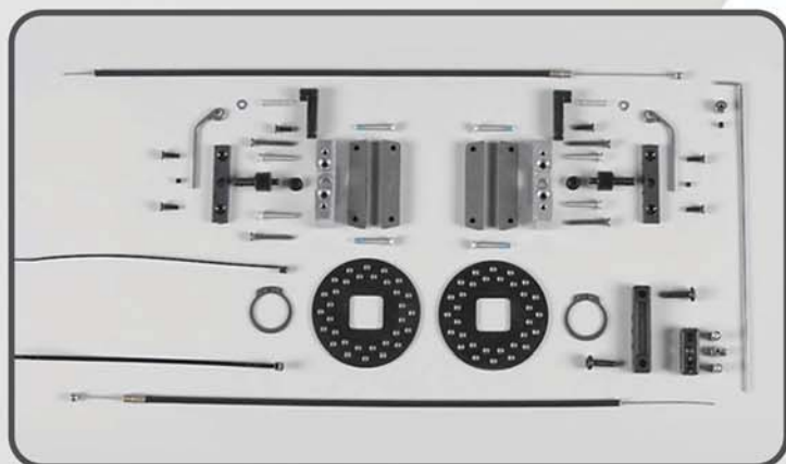
Scheibenbremse vorne für Monster, Set Front disk brake for Monster, set Freins à disque à l'avant pour Monster, kit Best.-Nr./ Item N°./ Réf. 06250/03
