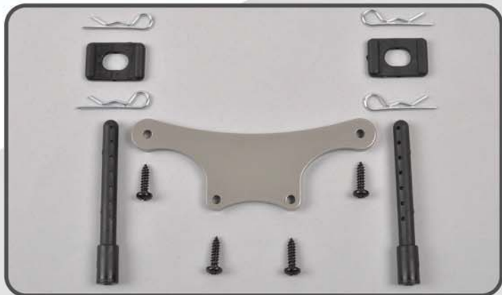
Aluminium Karosseriehalter vorne verstellbar, Set Aluminium body mounts front adjustable, set Supports réglables de carrosserie avant aluminium, kit Best.-Nr./ Item N°./ Réf. 04483/01
