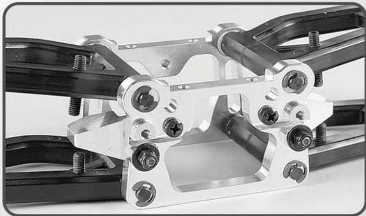
Alu-Vorderachsbock 2WD A und B Set Alum. front axle mount A and B set Cellule Av A + B alu, kit Best.-Nr./ Item N°./ Réf. 06496
