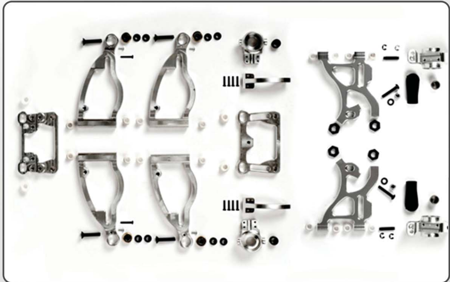
Legierung Umbausatz für Marder Alloy Conversion kit for Marder Kit de conversion en alliage pour Marder Best.-Nr./ Item N°/ Réf. 68515
