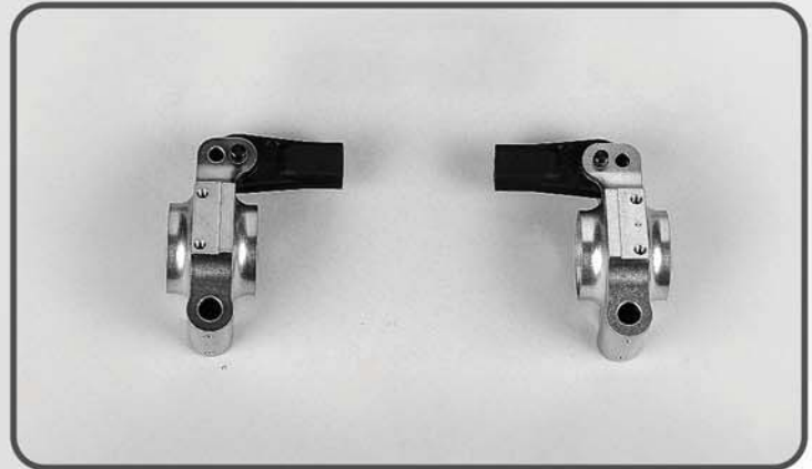
Alu-Achsschenkel hint. erhöht 1/6, Set Rear alum. uprights 1/6, raised, set Fusées arrière réhaussées alu 1/6, kit Best.-Nr./ Item N°./ Réf. 06478
