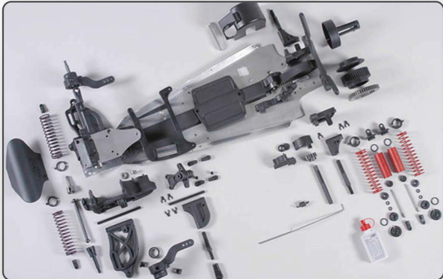
4WD Umrüstsatz für 2WD Marder in 4WD 4WD conversion kit for Marder 2WD to 4WD Kit de conversion pour Marder 2WD en 4WD Best.-Nr./ Item N°/ Réf. 68501
