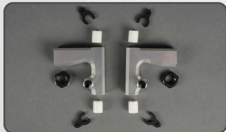
Alu-Querlenker hinten oben Set, 2 St. Rear upper aluminium wishbones set, 2 pcs. Kit de triangles aluminium arrière supérieurs, 2 pcs. Best.-Nr./ Item N°./ Réf. 04474
