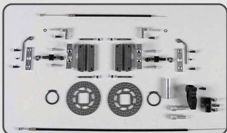
Tuning-Scheibenbremse hi. 1:5 Sportsline, Set Rear Tuning disk brake 1:5 Sportsline, set Frein à disque tuning arrière 1/5 Sportsline, kit Best.-Nr./ Item N°./ Réf. 08452/05
