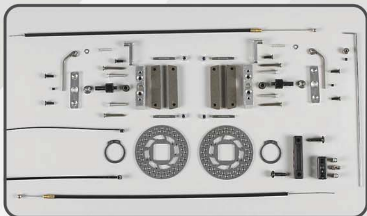
Tuning-Scheibenbremse vorne 1:6/2WD Monster-Modelle, 4WD Buggy, Set Front Tuning disk brake 1:6/2WD Monster models, 4WD Buggy, set Freins à disque tuning avant 1/6, modèles Monster 2WD, Buggy 4WD, kit Best.-Nr./ Item N°./ Réf. 06250/07
