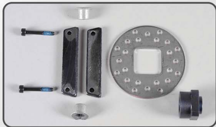
Tuning-Bremsset für Bremse 97, Set Tuning brake set for brake 97, set Kit de frein Tuning pour Frein 97 Best.-Nr./ Item N°./ Réf. 08449
