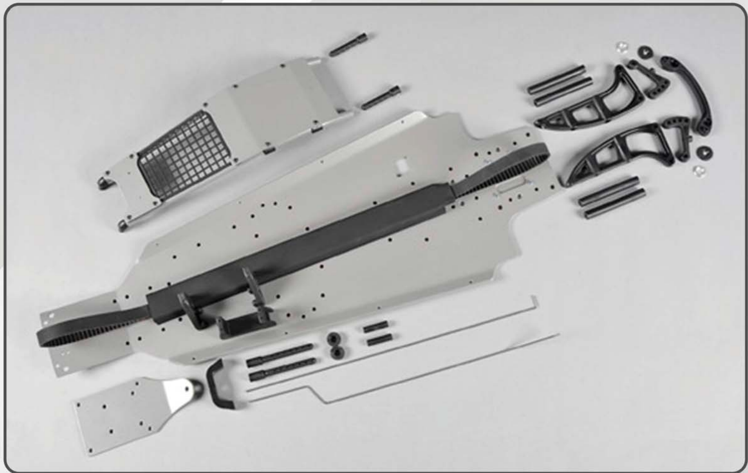
Umrüstsatz Off-Road Buggy 4WD auf 4WD WB535 Conversion kit Buggy WB535 Kit de conversion WB535 Best.-Nr./ Item N°/ Réf. 68532
