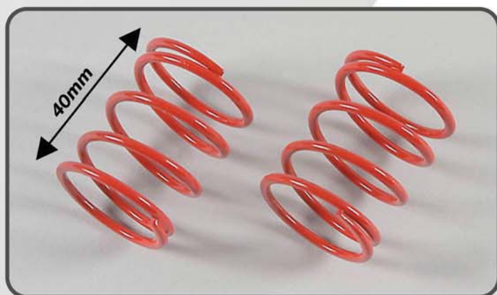
Dämpferfeder rot 2,5x40mm, 2St. Damper spring red 2,5x40mm, 2 pcs. Ressort d'amortisseur rouge 2,5x40mm, 2 pces. Best.-Nr./ Item N°./ Réf. 67313
