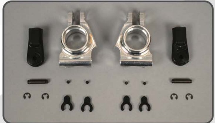
Alu-Achsschenkel hinten 1/5 und 1/6, Set Rear alum. uprights 1/5 and 1/6, set Fusées arrière aluminium 1/5 et 1/6, kit Best.-Nr./ Item N°./ Réf. 06477
