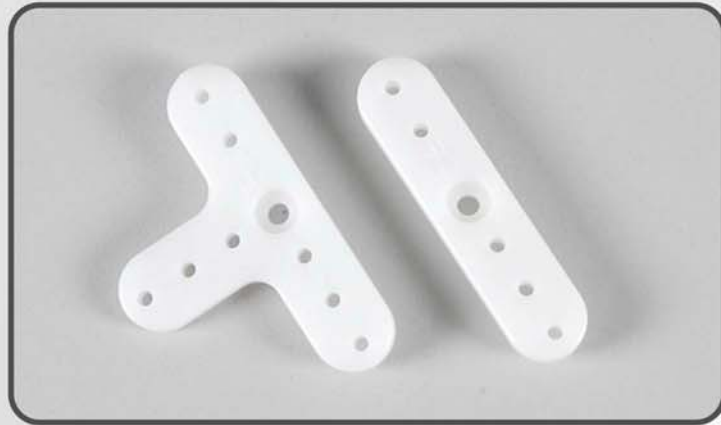
Servohebel JR/ MPX, 2 St. Servo arms JR/ MPX, 2 pcs. Palonniers JR/MPX, 2 pcs Best.-Nr./ Item N°./ Réf. 06536
