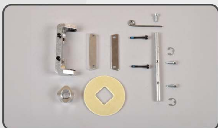
Bremse hinten 97 für 1/5 und 1/6 Rear brake 97 for 1/5 and 1/6 scale Frein de transmission 97 pour 1/5 et 1/6 Best.-Nr./ Item N°./ Réf. 07497
