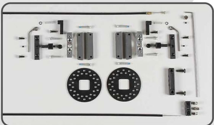
Scheibenbremse hinten F-1/5, Set Rear disk brake F-1/5, set Frein à disque arrière F-1/5, kit Best.-Nr./ Item N°./ Réf. 10451
