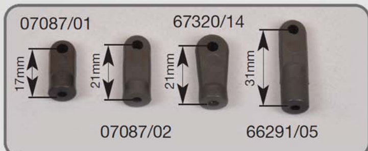
Dämpferbefestigungen Lower shock retaining Châpes d'amortisseur Best.-Nr./ Item N°./ Réf. 07087/01 2 pcs Best.-Nr./ Item N°./ Réf. 07087/02 2 pcs Best.-Nr./ Item N°./ Réf. 67320/14 4 pcs Best.-Nr./ Item N°./ Réf. 66291/05 2 pcs
