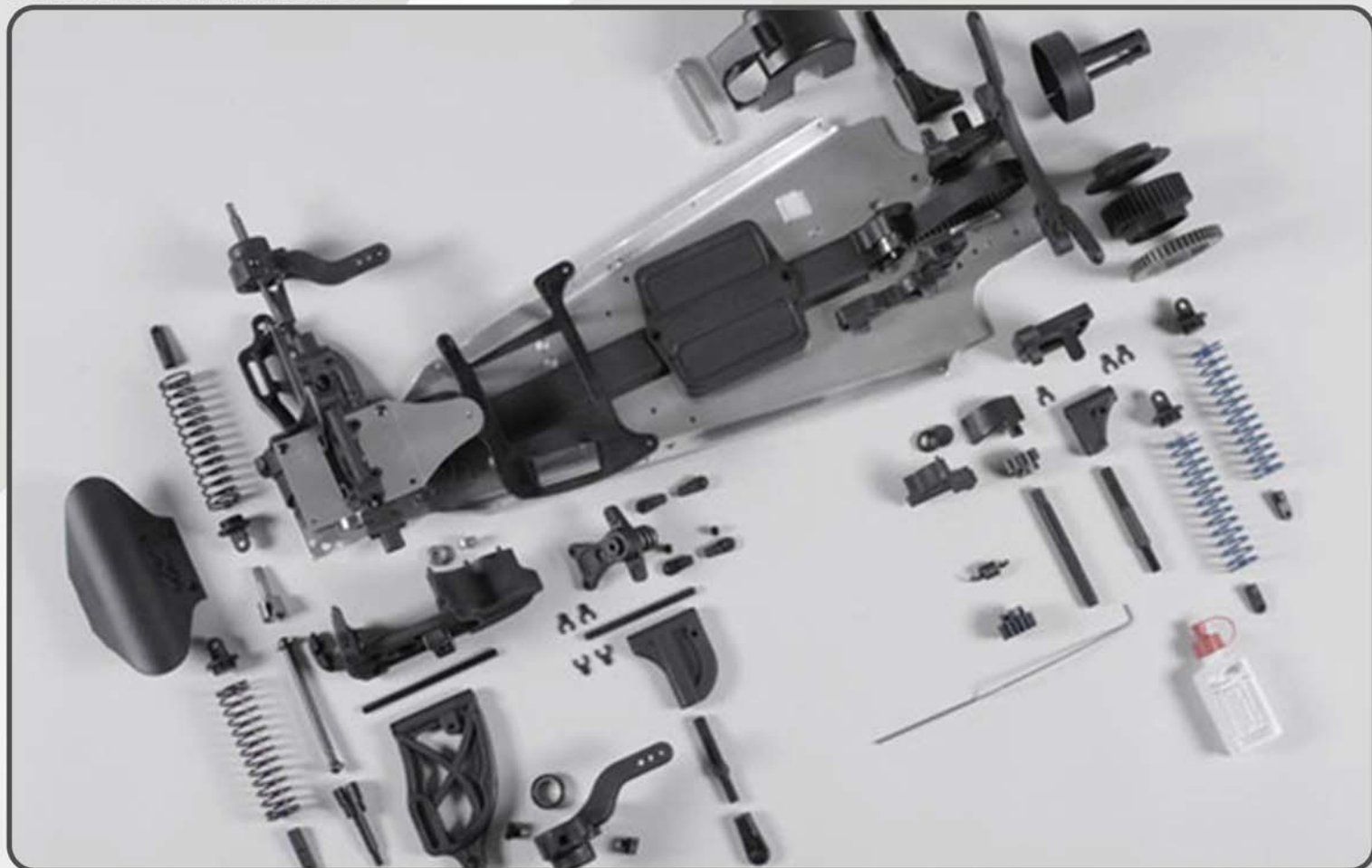
4WD Umrüstsatz für 2WD Monster 4WD conversion kit for Monster 2WD Kit de conversion 4WD pour Monster 2WD Best.-Nr./ Item N°/ Réf. 68500
