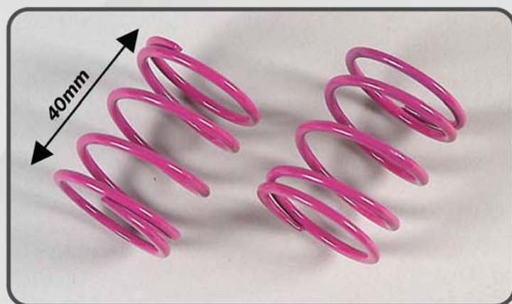
Dämpferfeder rosa 2,6x40mm, 2St. Damper spring pink 2,6x40mm, 2 pcs. Ressort d'amortisseur rose 2,6x40mm, 2 pces. Best.-Nr./ Item N°./ Réf. 67314
