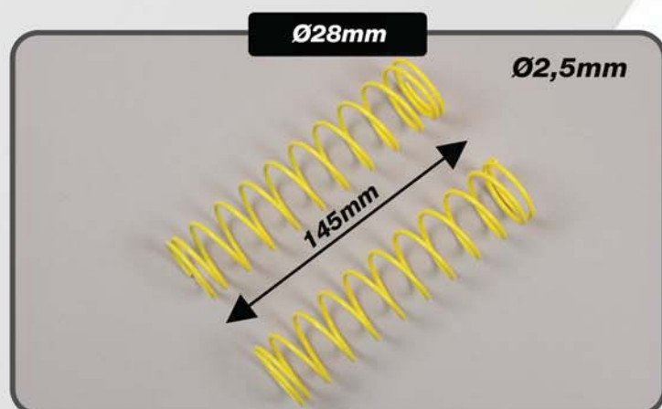
Stoßdämpferfeder, 2St. Damper spring, 2 pcs Ressorts, 2 pcs. Best.-Nr./ Item N°./ Réf. 67316
