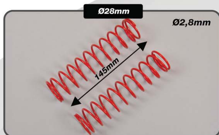
Stoßdämpferfeder, 2St. Damper spring, 2 pcs Ressorts, 2 pcs. Best.-Nr./ Item N°./ Réf. 67317
