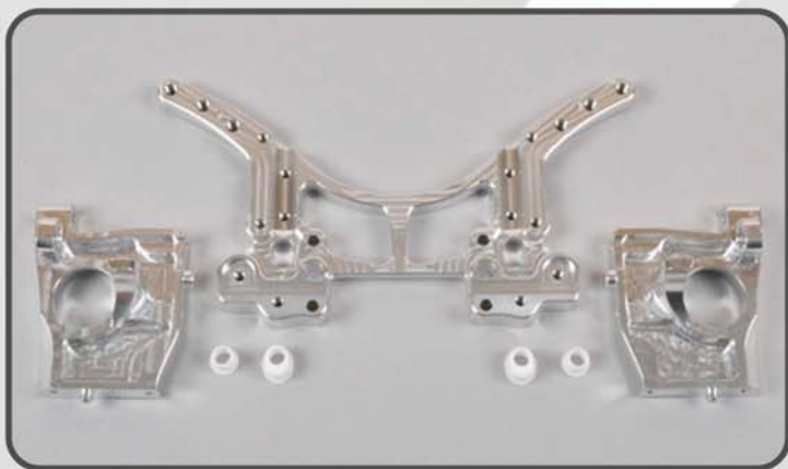
Alu-Dämpferplatte/-Hinterachsböcke, Set Alum. damper plate/ alum. rear axle mounts, set Supports amortisseurs/train arrière alu, kit Best.-Nr./ Item N°./ Réf. 68400/01
