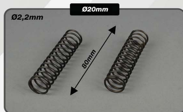
Stoßdämpferfeder, 2St. Damper spring, 2 pcs Ressorts, 2 pcs. Best.-Nr./ Item N°./ Réf. 06095
