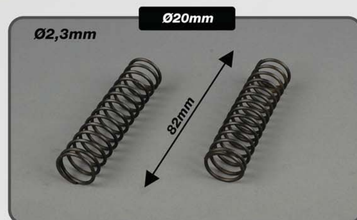
Stoßdämpferfeder, 2St. Damper spring, 2 pcs Ressorts, 2 pcs. Best.-Nr./ Item N°./ Réf. 06094/03
