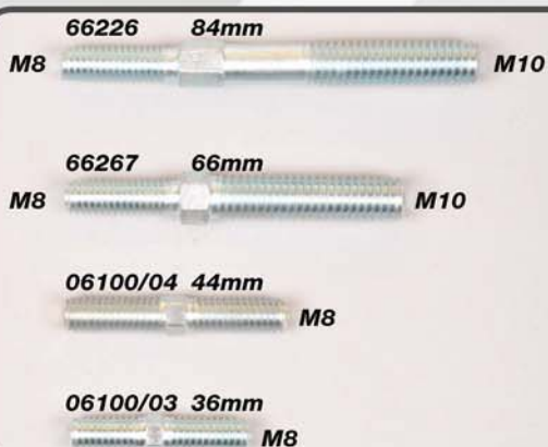
Stahl Querlenkergewindestangen Steel wishbone thread rod Pas inversés en acier Best.-Nr./ Item N°./ Réf.
