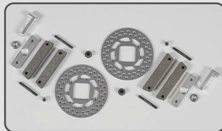
Umrüstset auf Tun.-Scheibenbr. vo/hi., Set Conversion kit to Tuning disk brake f./r., set Set de conversion frein à disque tun. AV/AR, kit Best.-Nr./ Item N°./ Réf. 06250/08
