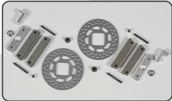
Umrüstset auf Tun.-Scheibenbremse vo/hi., Set Conversion kit to Tuning disk brake f./r., set Set de conversion frein à disque tun. AV/AR, kit Best.-Nr./ Item N°./ Réf. 08450/08
